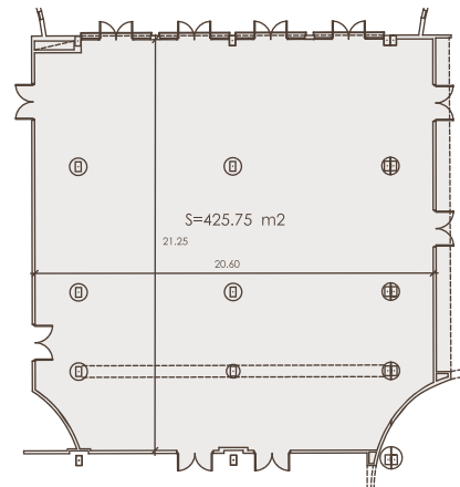
planta 0 E-1:150
